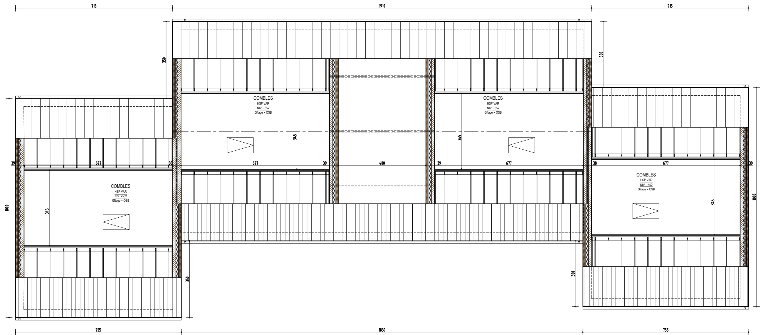
PLAN DES COMBLES
